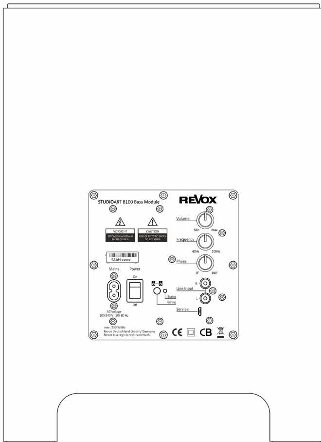
Rückansicht B100
