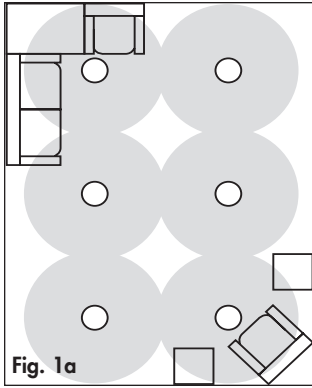
MC4/6/8: Haut-parleurs multiples, audio distribué.
