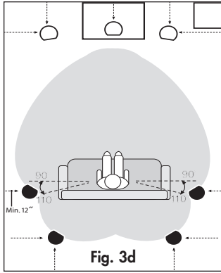
MC6-HT: Canaux surround et arrière à rayonnement direct dans un système à 7,1 canaux.
