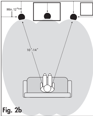
MC6-HT: Haut-parleurs avant gauche, central et droit.
