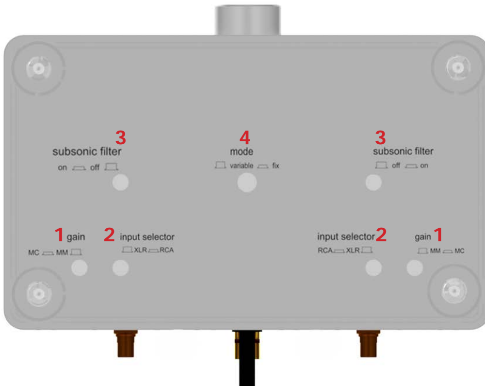
Abb. 1: Ansicht Bodenplatte der Phonovorstufe
